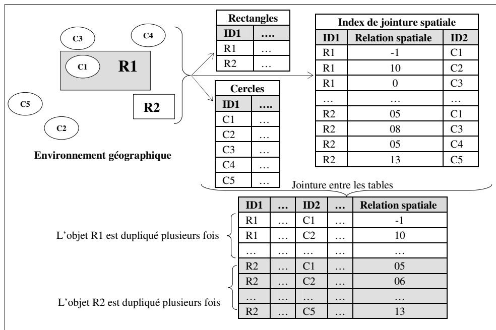
FIG 2: Index de jointure spatiale (en haut) et problème de la jointure (en bas).
