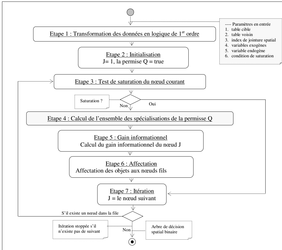
FIG 3: L'algorithme S-TILDE.
